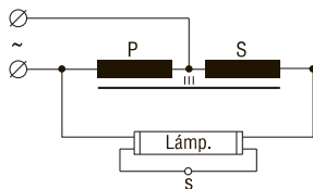
Autotransformador de dispersión Leakage autotransformer
