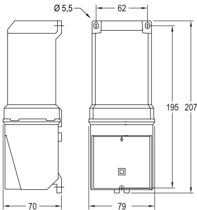
IP40 ASSEMBLIES WITH CONNECTION TERMINALS / EQUIPOS IP40 CON BORNES DE CONEXIÓN
