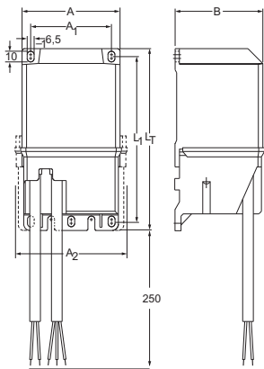
WITH COMMAND WIRES / CON LÍNEA DE MANDO
