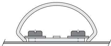
Diffuser fixing with M4 insulation ring Fijación del difusor mediante arandela de plástico M4 (Ref. 9710107 DIN-125 M4 x \varnothing 4,30 x \varnothing 9 x 0,80 6.6PA)
