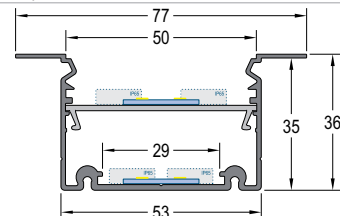
Blue rectangle shows the space for the LED strip El rectángulo azul muestra el espacio para la tira de LED
