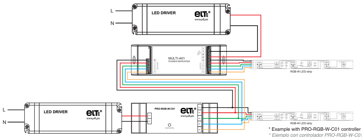
Connection diagram* Esquema de conexión*
